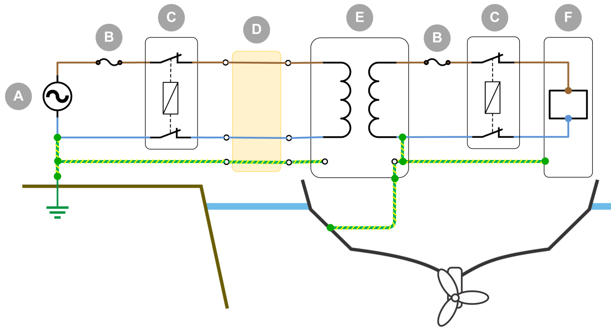
Johdotusesimerkki maasähköön kytketyn aluksen eristysmuuntajan asennuksesta.
